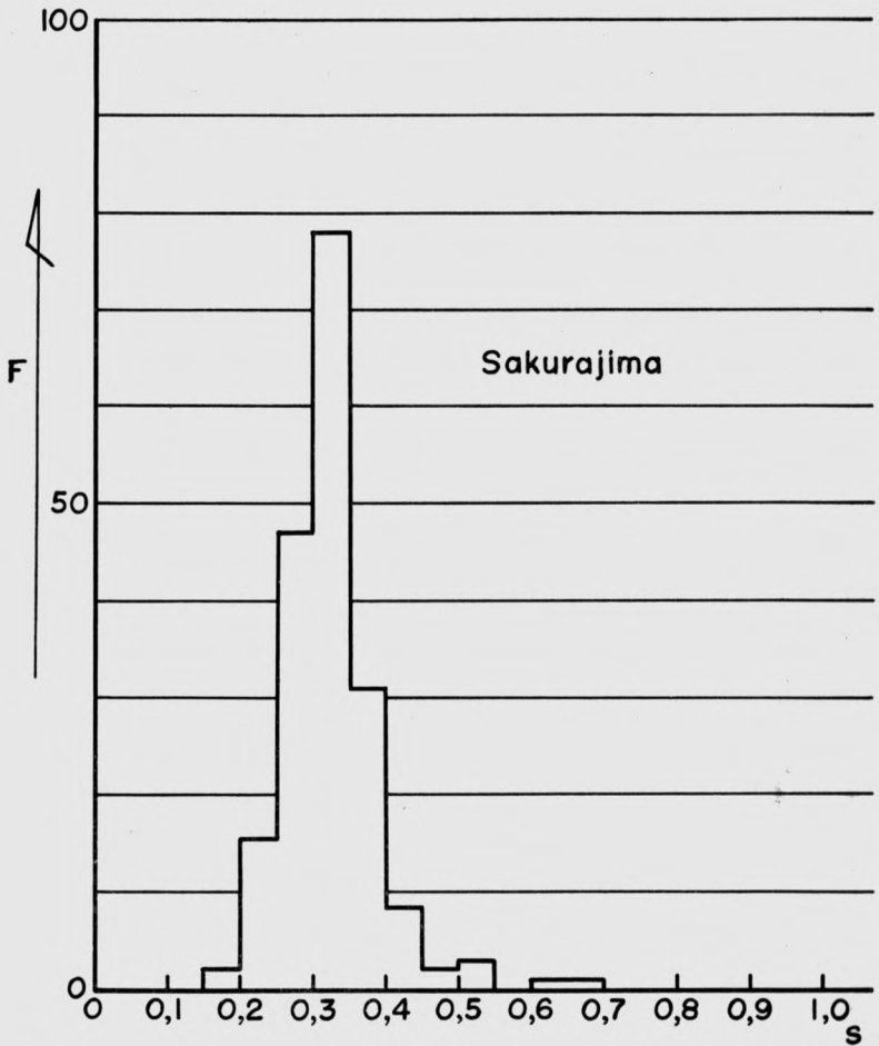
FIG. 8. — Distribution des fréquences des microséismes volcaniques observés à l'aide d'un séismographe horizontal au Sakura-zima (d'après MINAKAMI).
