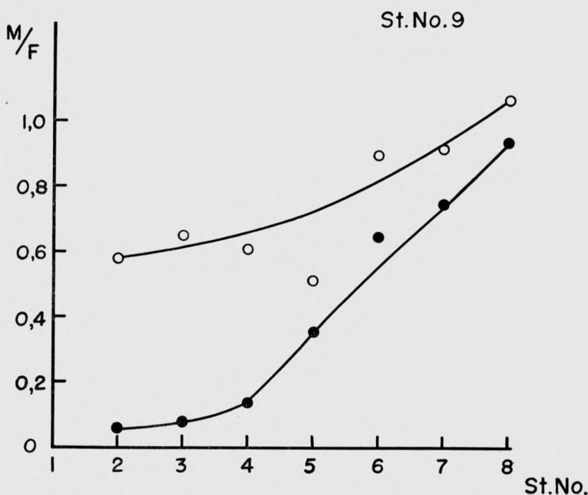
FIG. 16. — Facteur d'amplitude des stations de la plate-forme supérieure par rapport à la station n° 9.
