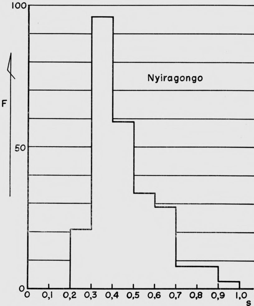
FIG. 5. — Distribution des fréquences des microséismes volcaniques observés par séismographe horizontal au Nyiragongo.
