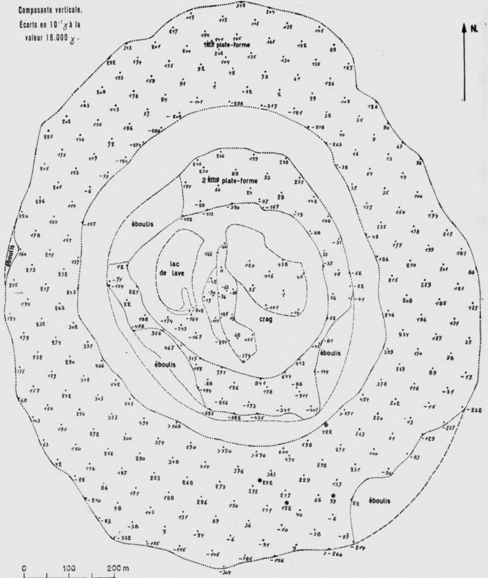
FIG. 5. — Valeurs des anomalies de Z, en dizaines de \gamma , à l'intérieur du cratère.
