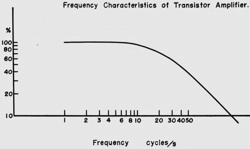
FIG. 2. — Caractéristiques de fréquence de l'amplificateur à transistors.
