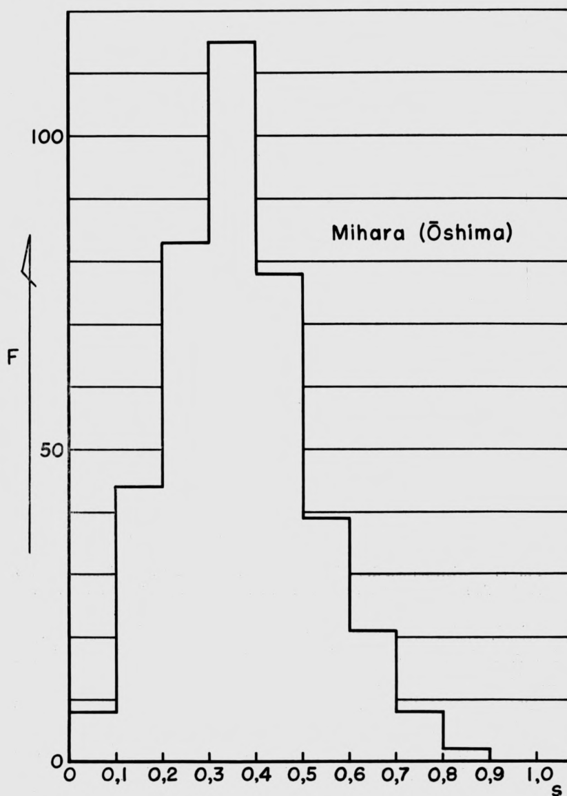
FIG. 7. — Distribution des fréquences des microséismes volcaniques observés à l'aide de séismographe horizontal au Mihara (d'après MINAKAMI).
