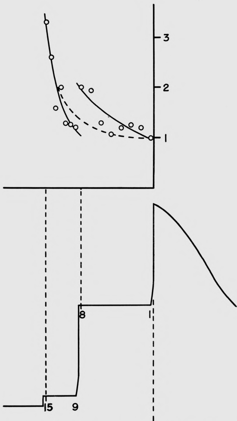
FIG. 15. — Amplitude relative sur les plates-formes supérieure et inférieure près de la station n° 1 en correspondance avec la section verticale du cratère.
