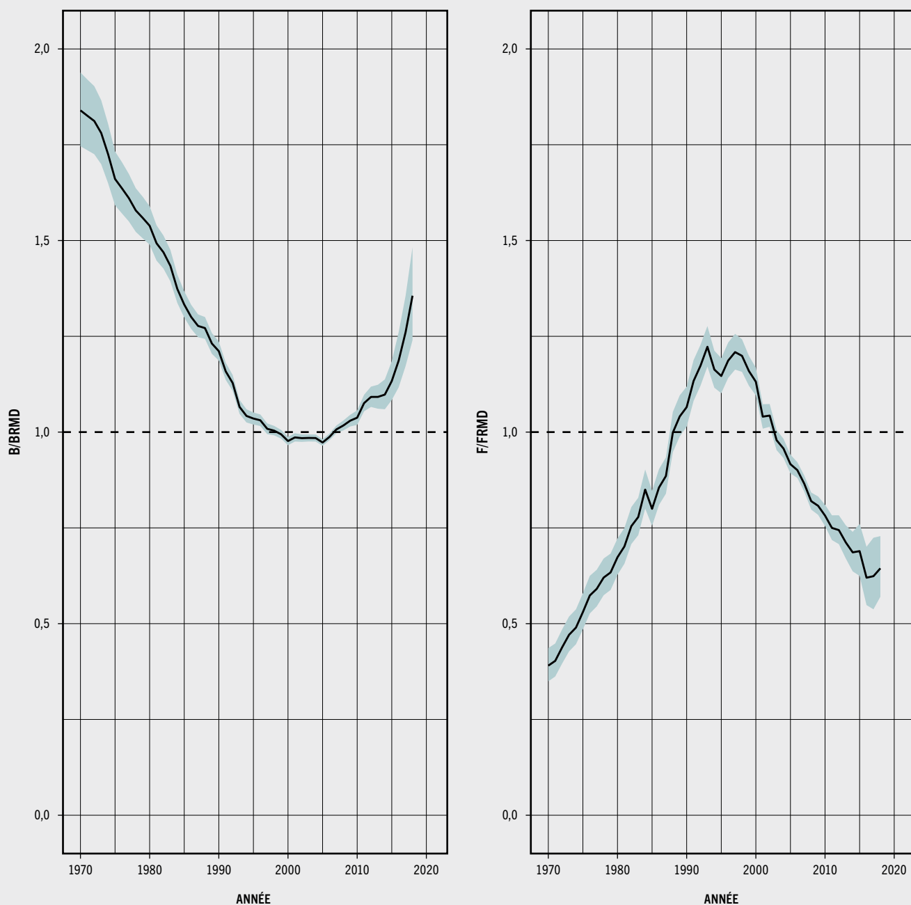
FIGURE B TENDANCES MONDIALES DE LA BIOMASSE RELATIVE (B/BRMD) DES STOCKS ÉVALUÉS DE POISSONS ET D'INVERTÉBRÉS ET DE LA PRESSION DE PÊCHE RELATIVE (F/FRMD) ESTIMÉES SELON UN MODÈLE ESPACE-ÉTAT 1
