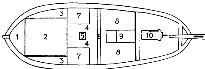
Na aanbrengen van den motor. 1 boeg, 2 „fronger”, 3 „zealkojen”, 4 „op 't ozes”, 5 mast, 6 „ozes”, 7 „eeskejen”, 8 „reum”, 9 „kot”, 10 motor.
