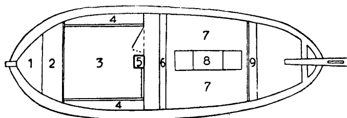
Botter zonder motor. 1 boeg, 2 gemeensch. {kooi, 3 „fronger”, 4 zeilbergplaatsen, 5 mast, 6 „ozes”, 7 „reum”, 8 „kot”, 9 „picke”.
