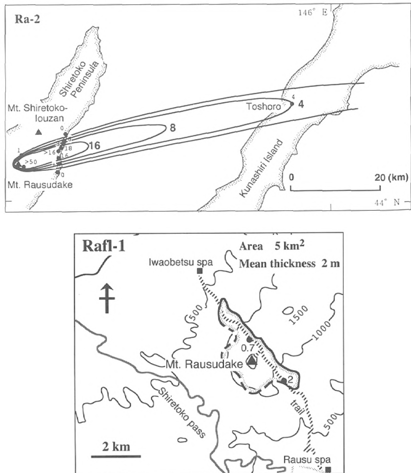
図 2-2 約 1400～1600 年前の噴火によるテフラ(上)および約 500～700 年前の噴火による火砕流分布(下)(宮地・他, 2000)
