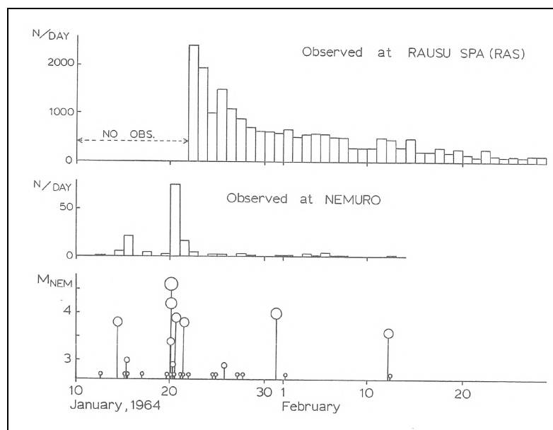
図 2-3 1964 年 1～2 月の日別地震発生数の推移 (上段：北大理学部による臨時観測の結果 中下段：根室測候所の資料) および地震活動経過図(勝井・他, 1982)
