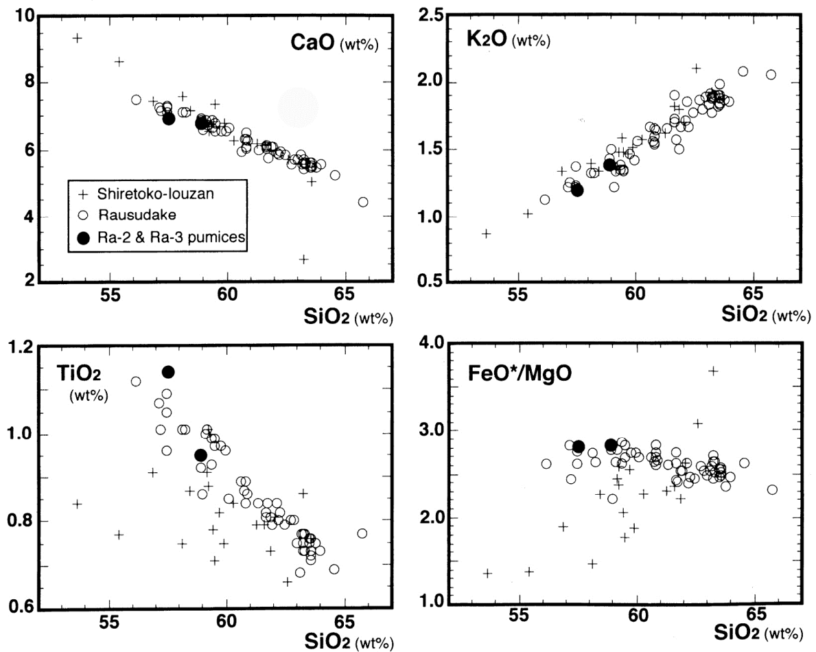
図 2-1 全岩化学組成ハーカ一図(宮地・他, 2000)
