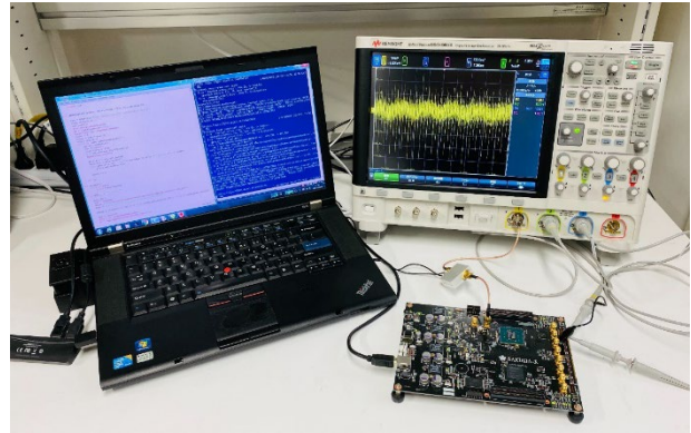
図 2: 開発した対策技術による安全性実証実験の様子: 物理的に観測されても PQC の動作中に秘密が漏えいしないことを実証
