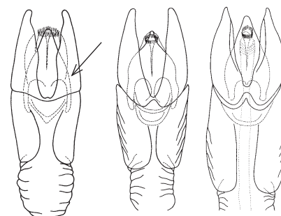
C. blanchardi C. semistriata C. toddi
