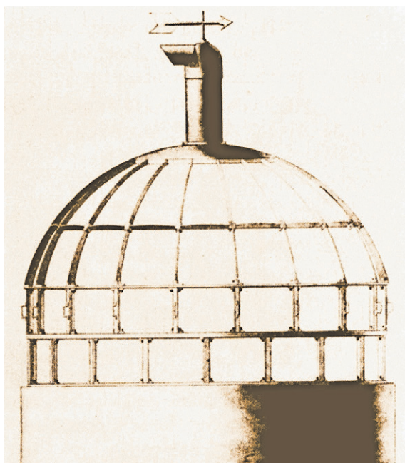
Entwurf Repsolds einer Laterne für den Leuchtturm Neuwerk um 1810.
